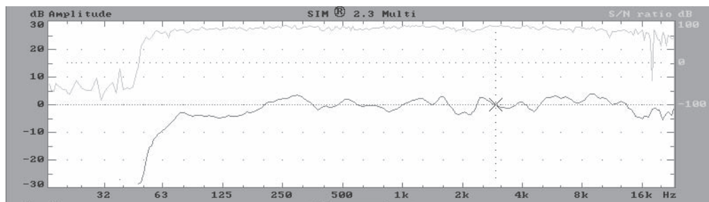
Fig 1.2e UPA-1C on-axis amplitude response.
