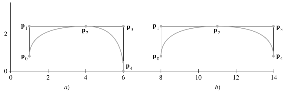
FIGURA 3 a) Continuidad G^1 y b) continuidad C^1 .
