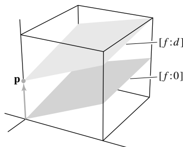
FIGURA 1 Hiperplanos paralelos, con f(\mathbf{p}) = d .
