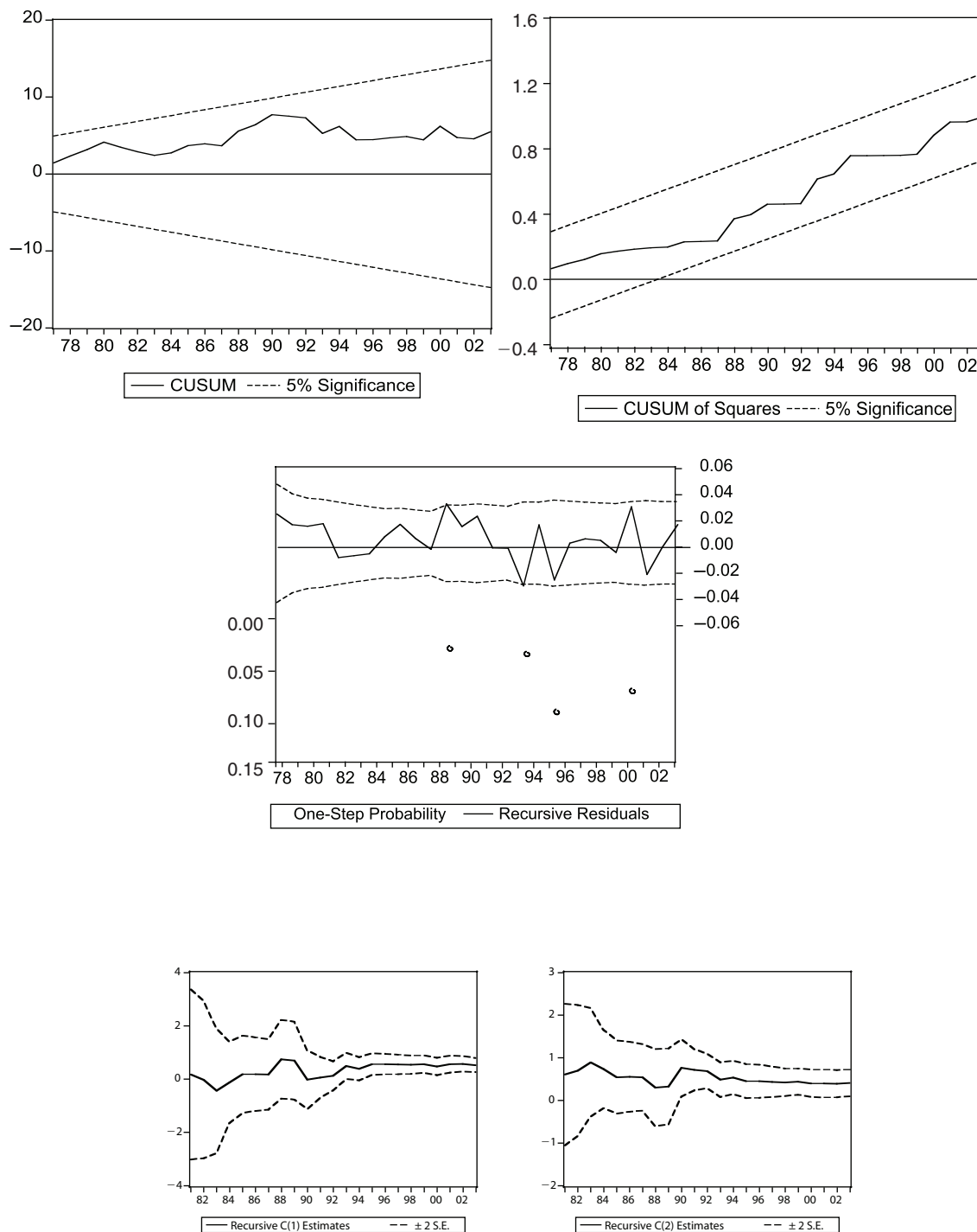
GRÁFICA 7.5 Pruebas de cambio estructural Consumo privado
