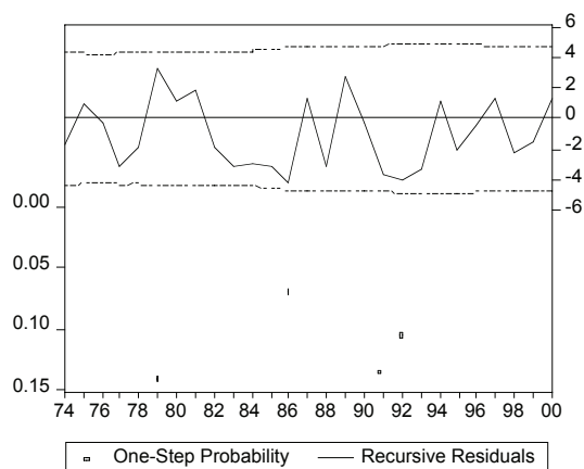
GRÁFICA 6.6 Prueba one-step de residuos
