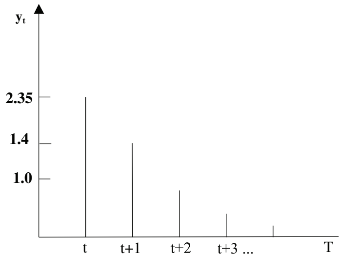
GRÁFICA 9.7 Efecto marginal (asintótico) del aumento de C_t
