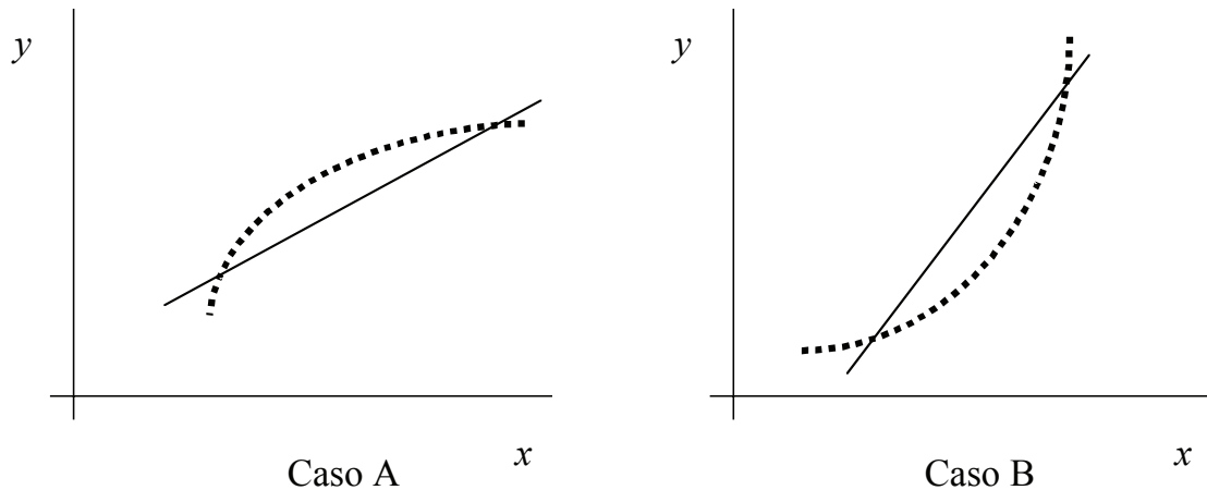
GRÁFICA 7.3 Forma funcional lineal-log
