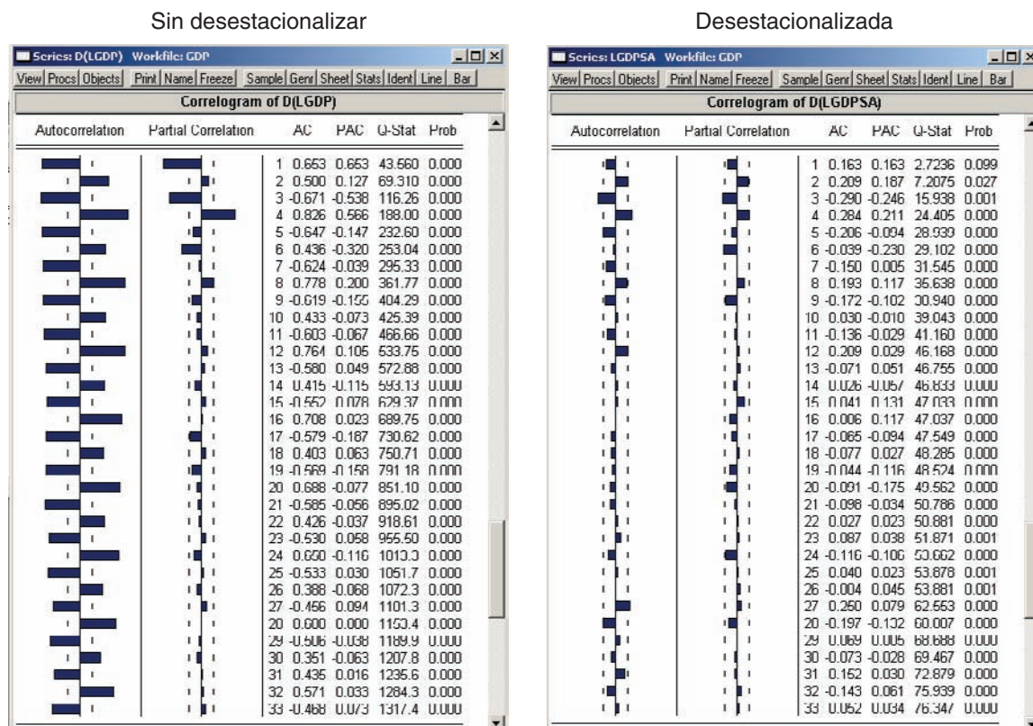
GRÁFICA 6.10 México: PIB observado y desestacionalizado 1980.1-2004.4
