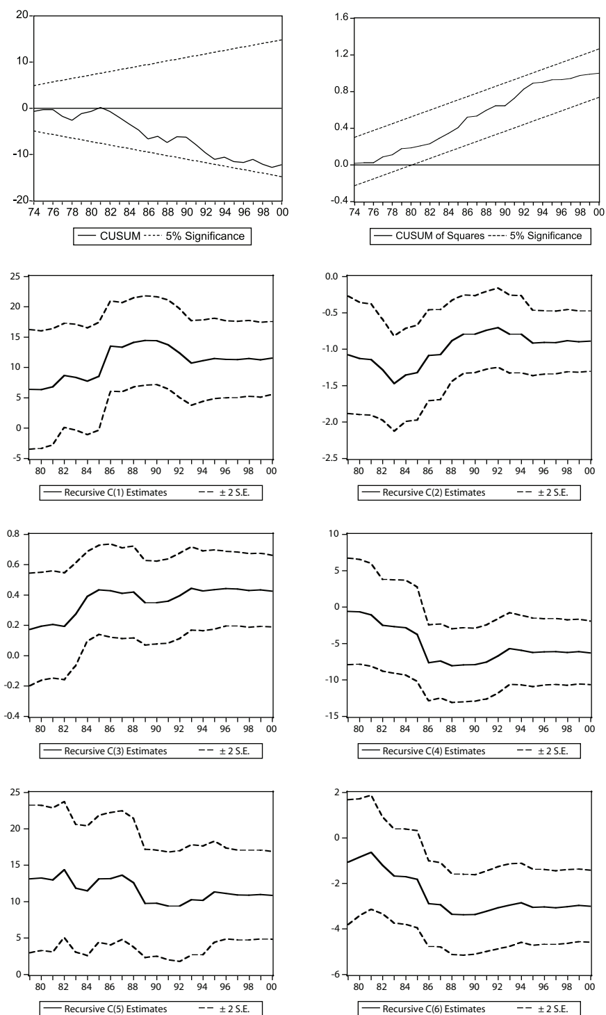
GRÁFICA 6.5 Modelo de ajuste parcial. Pruebas de estabilidad estructural y coeficientes recursivos
