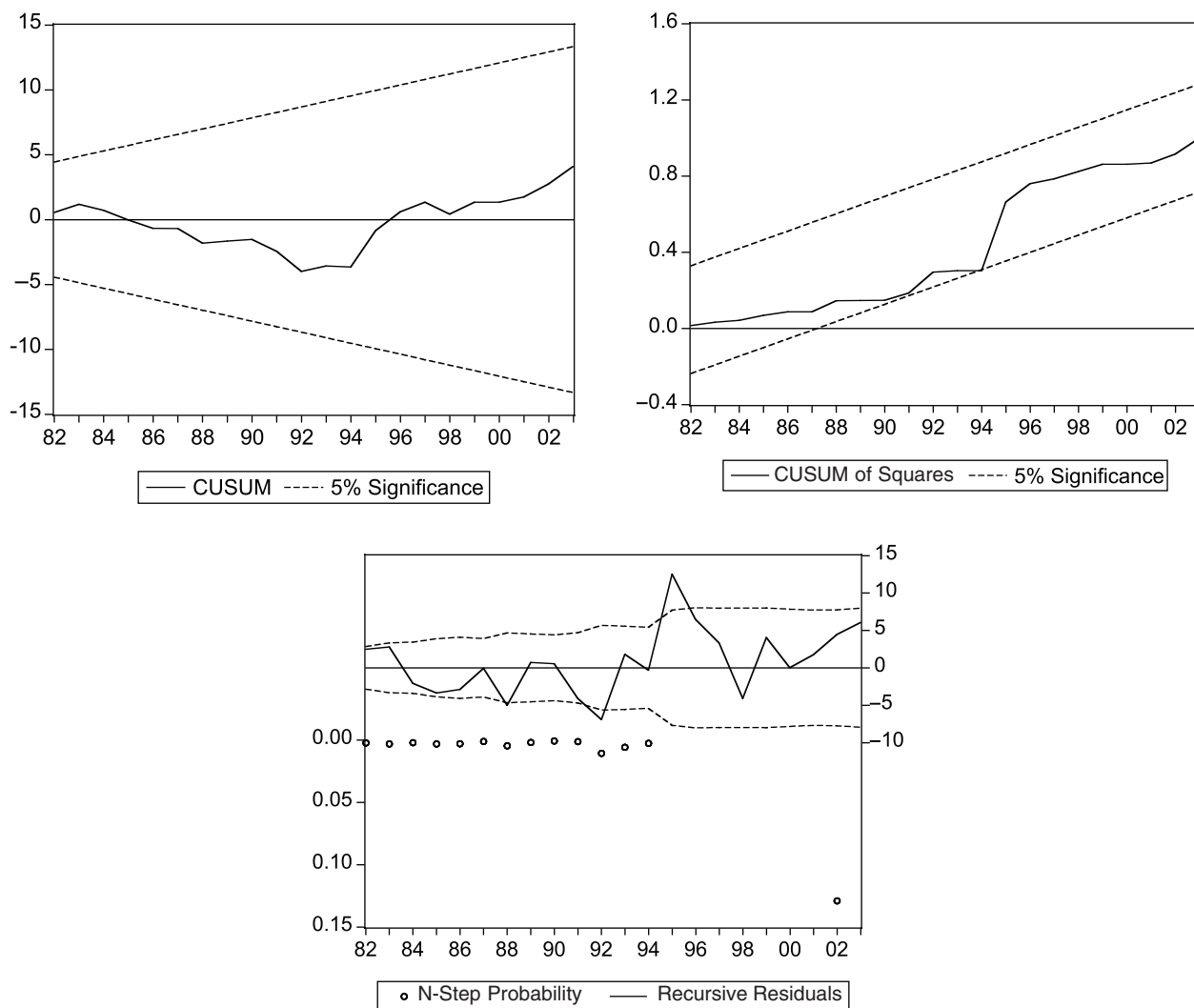
GRÁFICA 7.12 Pruebas de cambio estructural Cuenta corriente
