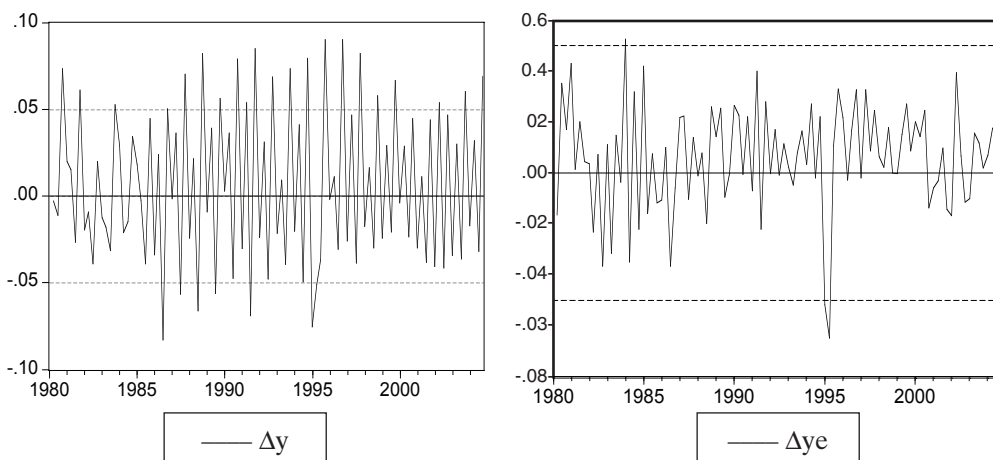
GRÁFICA 6.11 México: primera diferencia del PIB
