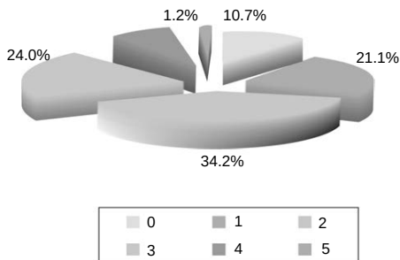
Figura 7–7. La prevalencia de SM en el Distrito Federal según la clasificación de la Federación Internacional de Diabetes (IDF), y de acuerdo al número de componentes del síndrome ( n = 6\,161 ), con esta clasificación la prevalencia global en D. F. es de 21.1 a 88% dependiendo la presencia de cada uno de ellos.
