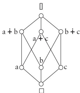
Figura 1.2 Semirretículo generado por S = \{\square, a, b, c, \square\} .
