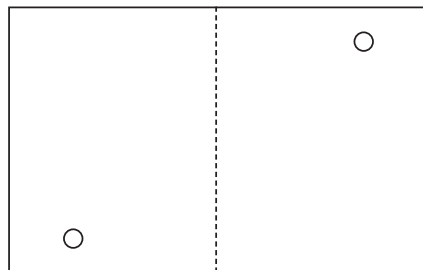
Figura 2.3. Dos electrones en una caja: intercambiables si están en el mismo estado, pero distintos y distinguibles (discernibles). O sea, el que los intercambiamos no tiene efecto sobre los estados del sistema como totalidad.
