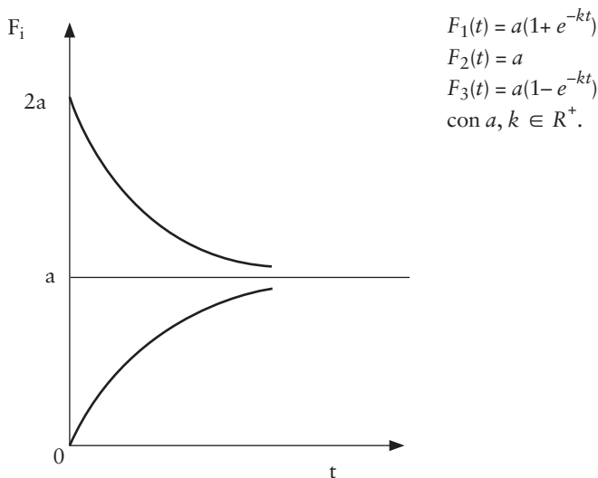
Figura 5.11. Tres modos diferentes de alcanzar el mismo estado final o valor asintótico X_\infty = a , aumentando hasta a o decreciendo hasta él.
