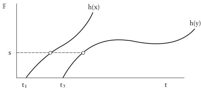
Figura 5.14. Cosas diferentes pueden ocupar el mismo estado, a condición de que lo hagan en instantes diferentes.
