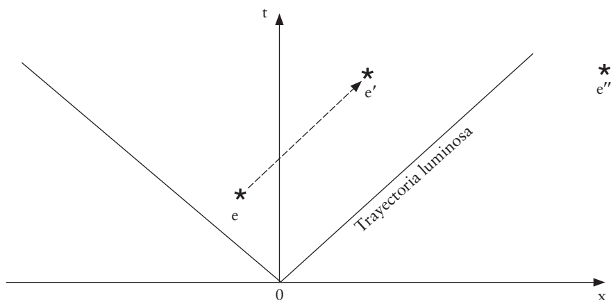
Figura 6.9. Sucesos e y e' son conectables, pero e y e'' no lo son, porque no hay señales superluminosas (conocidas).
