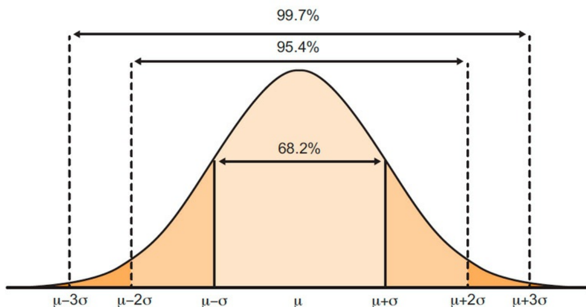
Figura 11-3. Porcentajes de área bajo la curva a distintas desviaciones estándar de la distribución normal.
