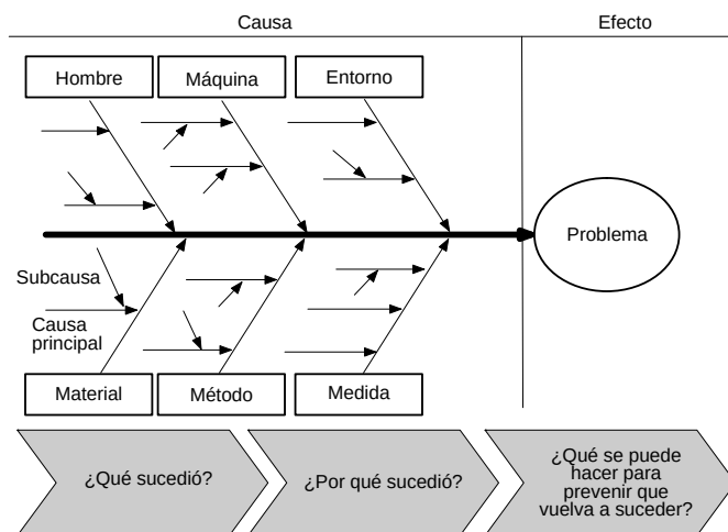
Figura 11–8. Diagrama causa-efecto.
